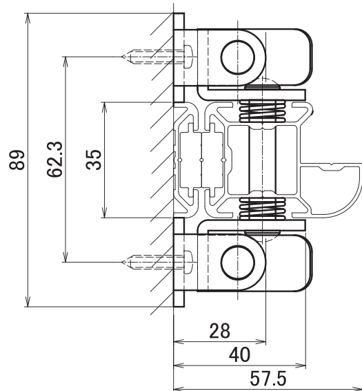
壁面 取付け
