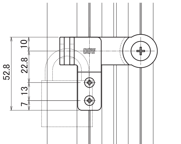
南京錠取付穴 \phi 10
